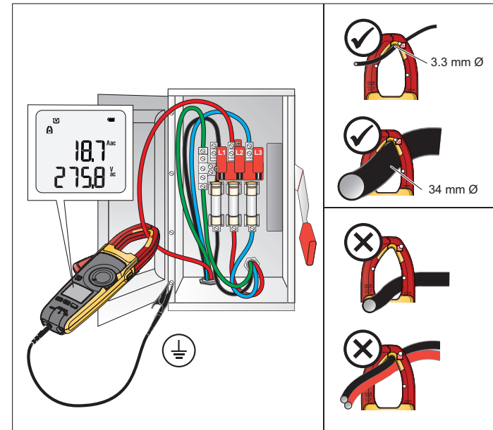
Figura 2. Colocación de los cables
