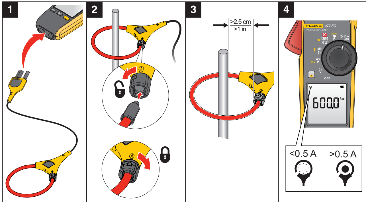
Figura 3. Configuración de la sonda iFlex
